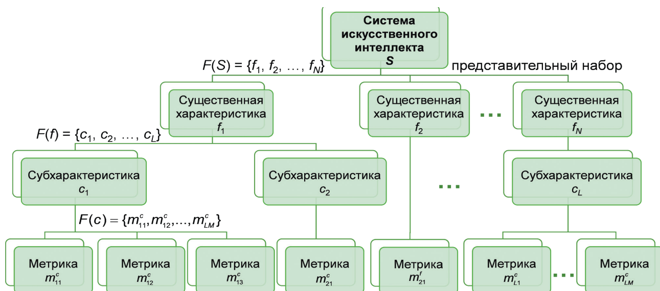
Рис. 1. Модель качества СИИ как продукта
